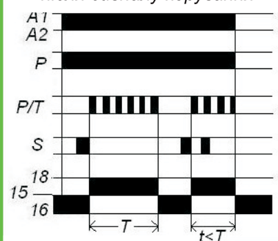
Функс G. Затримка відключення після сигналу керування
