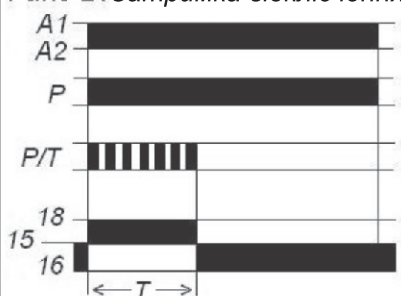
Функс Е. Затримка відключення після сигналу керування
