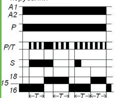
Функс H. Затримка відключення після затримки сигналу керування
