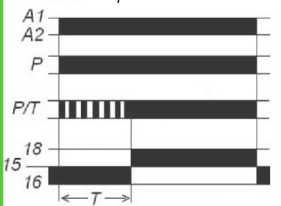
Функс D. Мультивібратор меандр починається з вкл.
