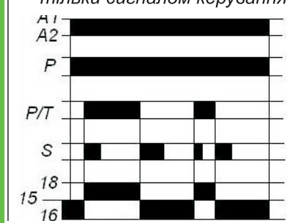
Функс I. Включення-відключення тільки сигналом керування
