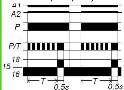
Функс J. Генератор імпульсу
