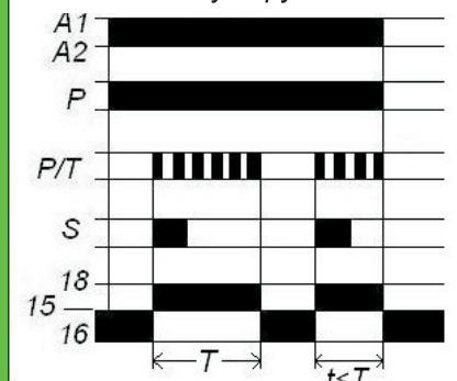
Функс I. Включення-відключення тільки сигналом керування
