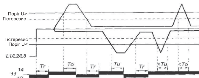
Діаграма роботи при підвищенні і зниженні Un
