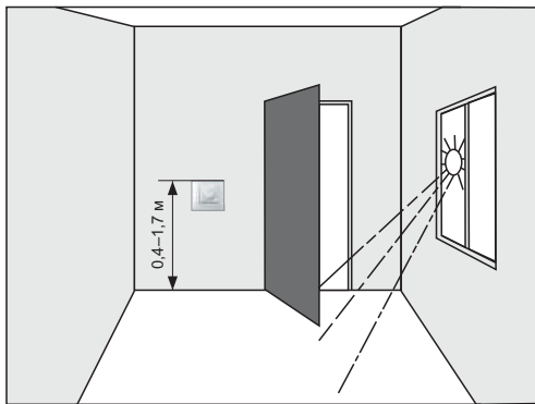
Рисунок 1. Монтаж терморегулятора монтом не больше 0,5 Н × м.
