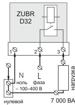
Схема 1. Упрощенная внутренняя схема и схема подключения
